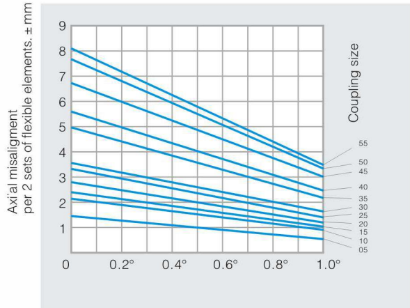
A-TYPE(4Bolt)
